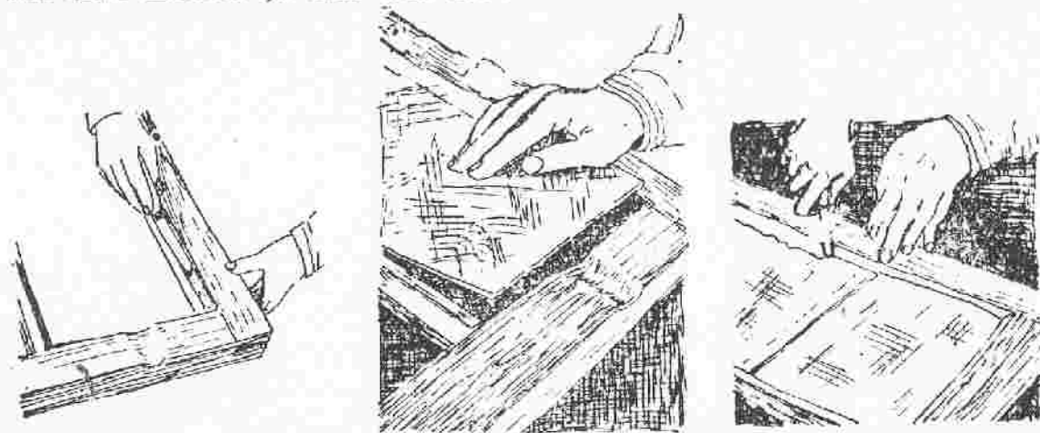
Zoon. 35. 1 — wana kitt eemaldatakse raami waltstist, 2 — uus klaas asetatakse waltsti, 3 — kitt tõmmatakse siledaks.
